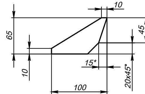
Поз.2 (Косынка)
