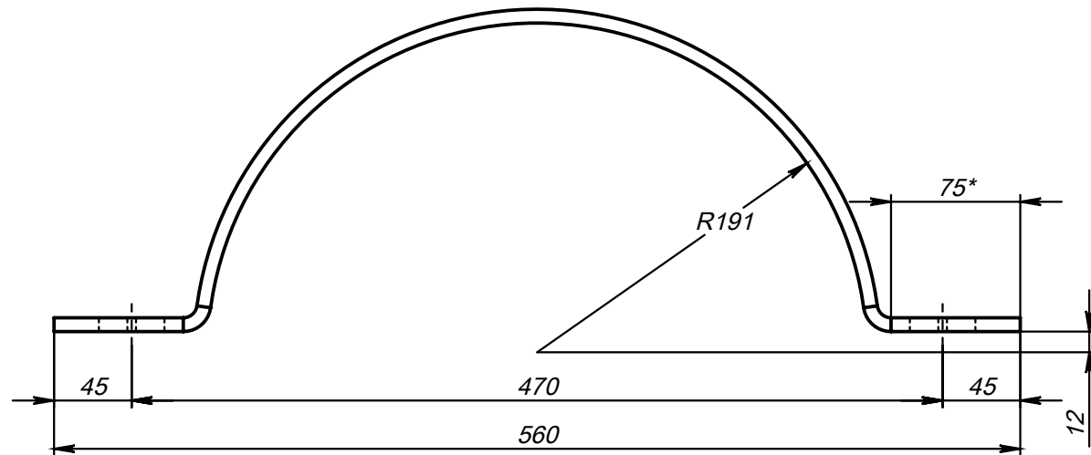
Поз.1 (Полухомут)
