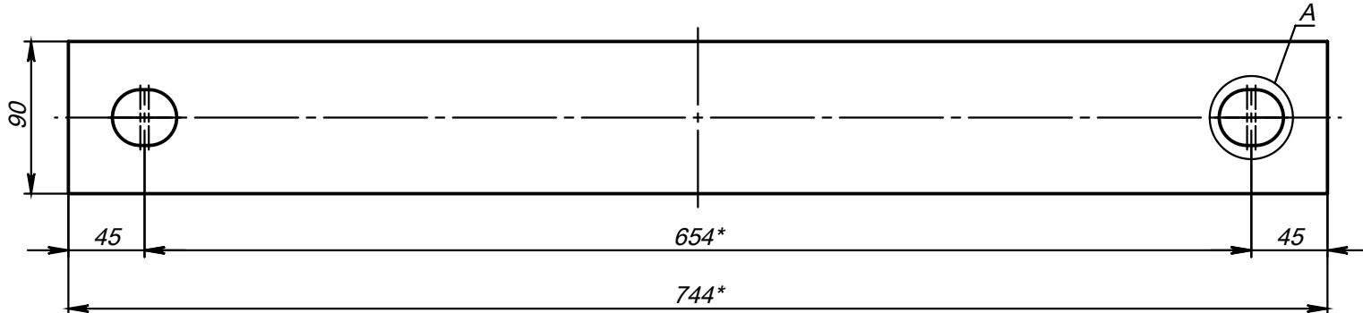
Поз.1 (Полухомут) развертка
